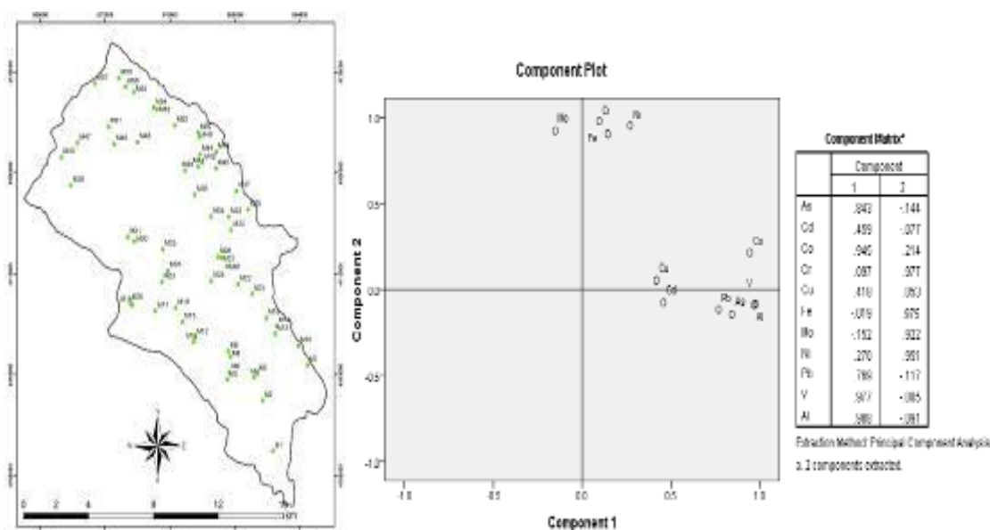
شکل ۷. نمودار تحلیل مولفه اصلی عناصر سنگین و موقعیت نقاط نمونه برداری شده در حوضه مطالعاتی؛ منبع: نگارندگان، ۱۴۰۱
