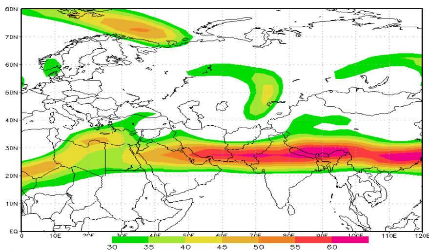
شکل ۱۰. موقعیت رودباده‌ها در روز ۲۷ مرداد ۱۳۸۱. منبع: نگارندگان، ۱۳۹۱
