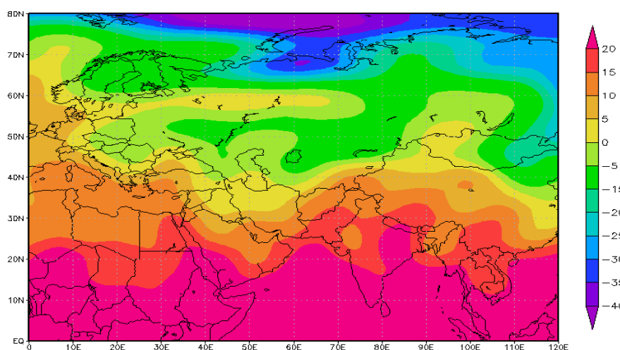
شکل ۷. توزیع دمای تراز دمای تراز ۱۰۰۰. منبع: نگارندگان، ۱۳۹۱
