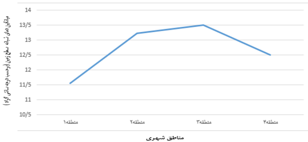
شکل ۱۲. روند تغییرات دمای شبانه سطح زمین مناطق ۱ تا ۴ بین سال های ۲۰۰۰ - ۲۰۲۲
