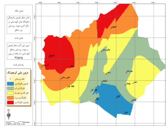
شکل ۵. درون‌یابی تأثیر منظر طبیعی بر هویت روستایی مناطق کوهستانی با استفاده از روش کریجینگ منبع: نگارندگان، ۱۳۹۶
