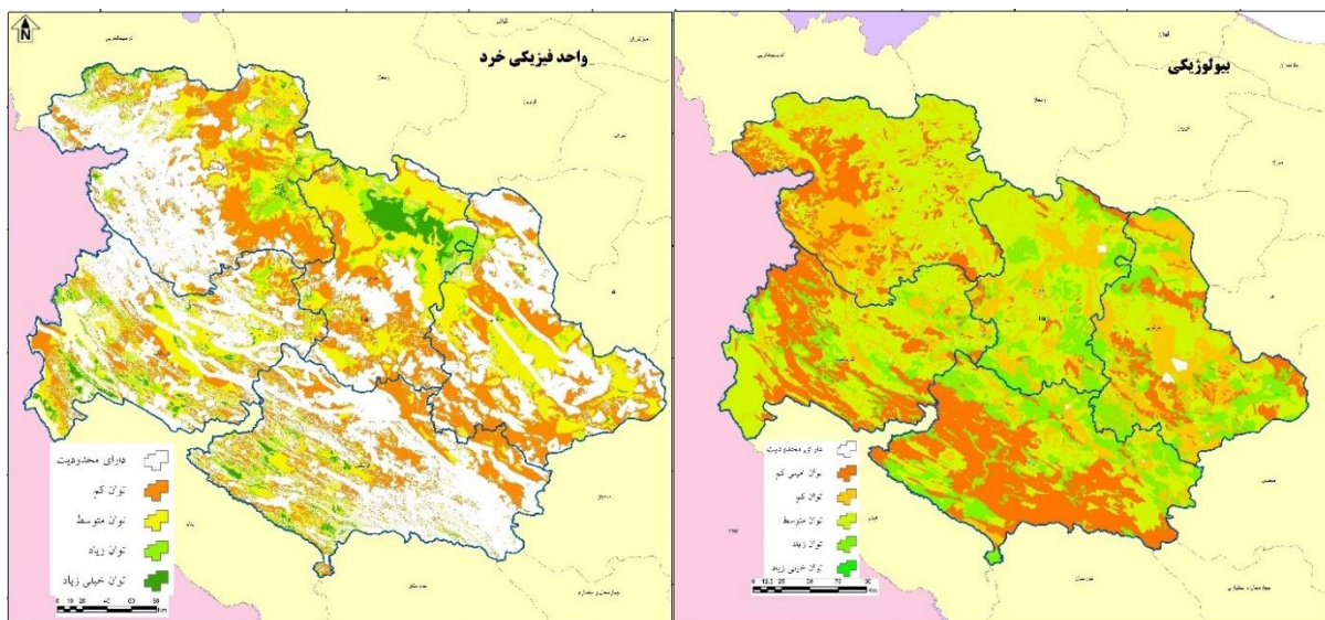
شکل ۳- نقشه واحد فیزیک خرد (چپ) و بیولوژیکی (راست) منبع: نگارندگان، ۱۴۰۰
